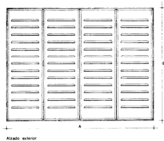
Alzado exterior
