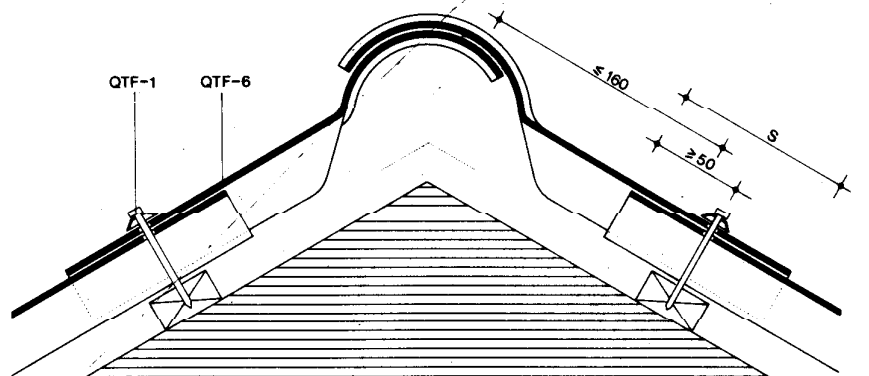
Fijación con tornillo
