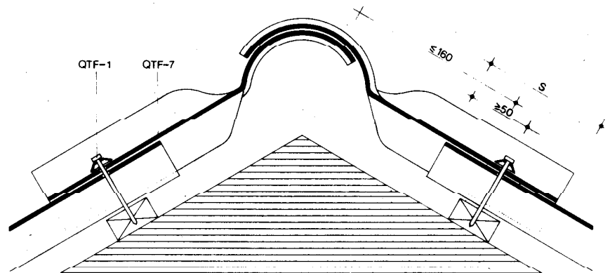
Fijación con tornillo
