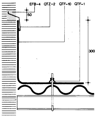
Fijación con gancho Sección
