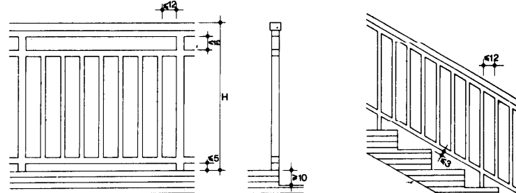
Viviendas y escuelas Alzado
